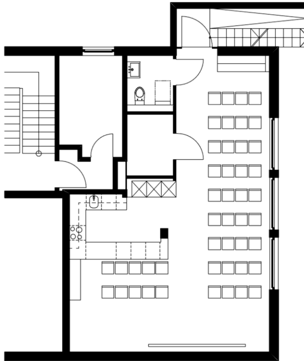
Reihenbestuhlung: 46 Plätze
